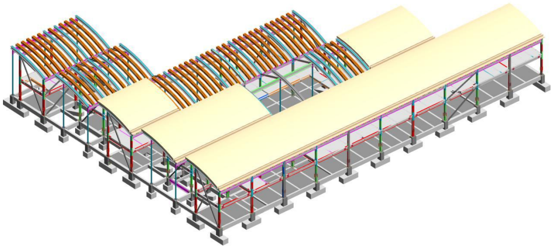
指挥部 BIM 模型
