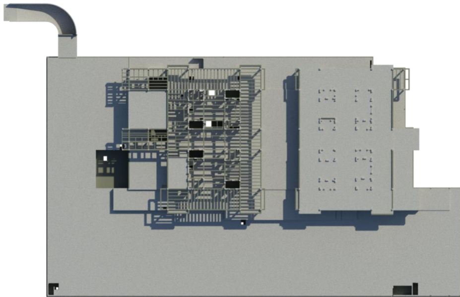
图书馆一层 BIM 模型
