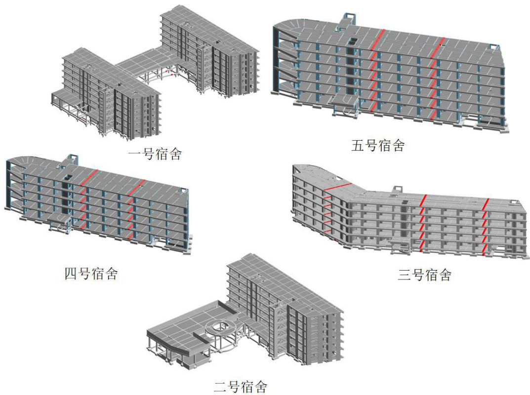
学生宿舍 BIM 模型
