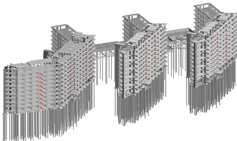
学生宿舍主体结构 BIM 模型
