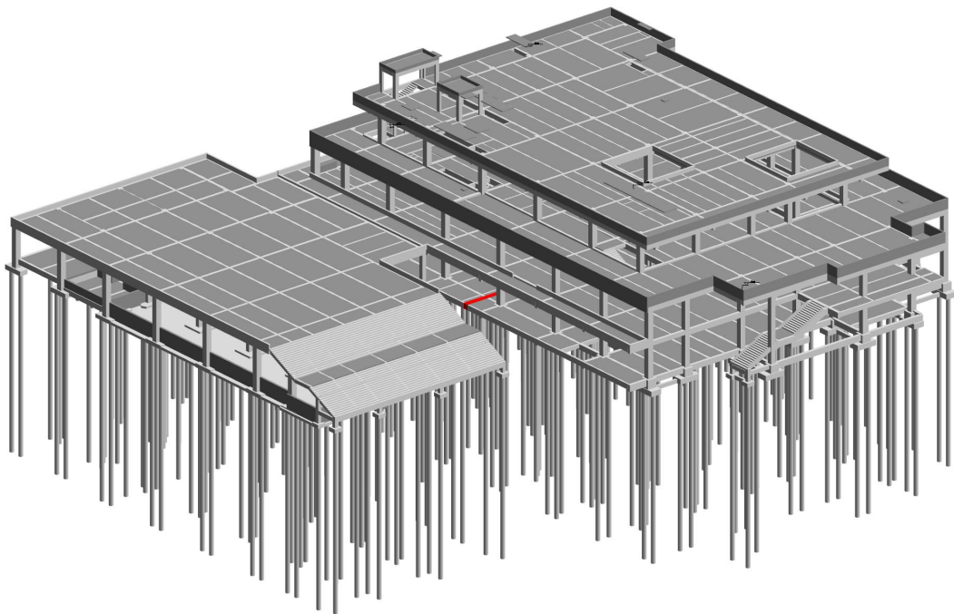
食堂（能源站）主体结构 BIM 模型
