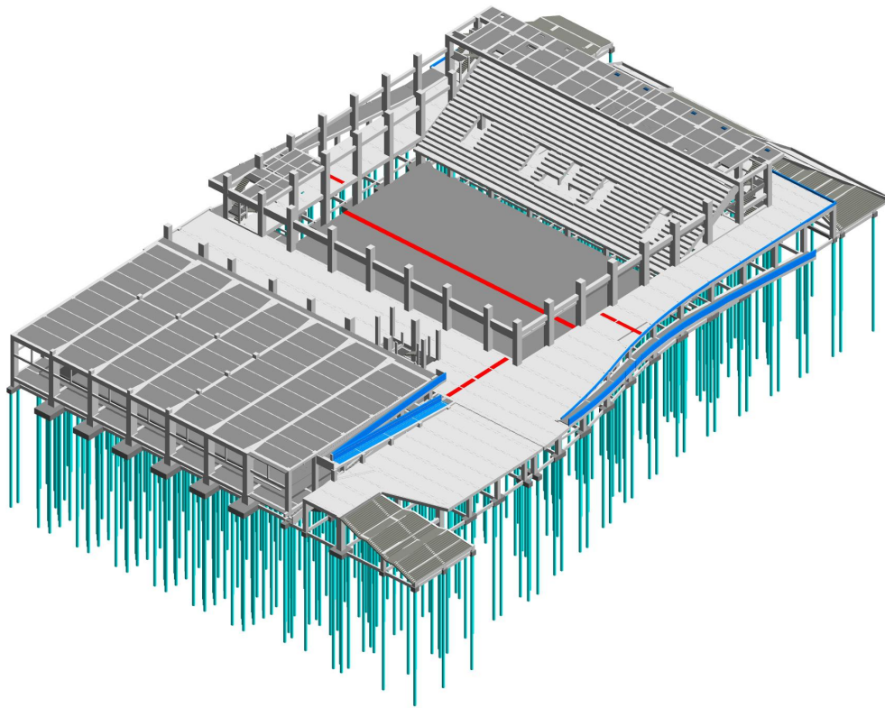
体育馆主体结构 BIM 模型
