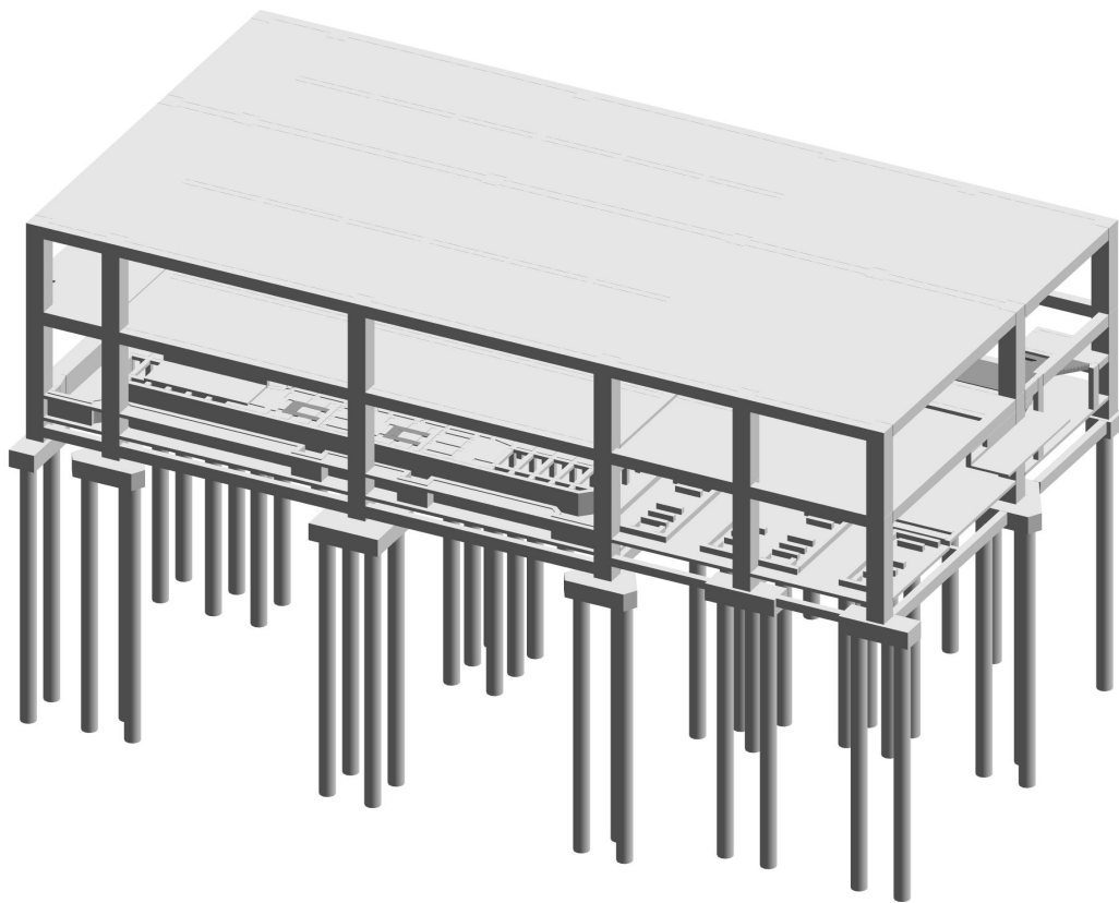
35KV 变电站 BIM 模型
