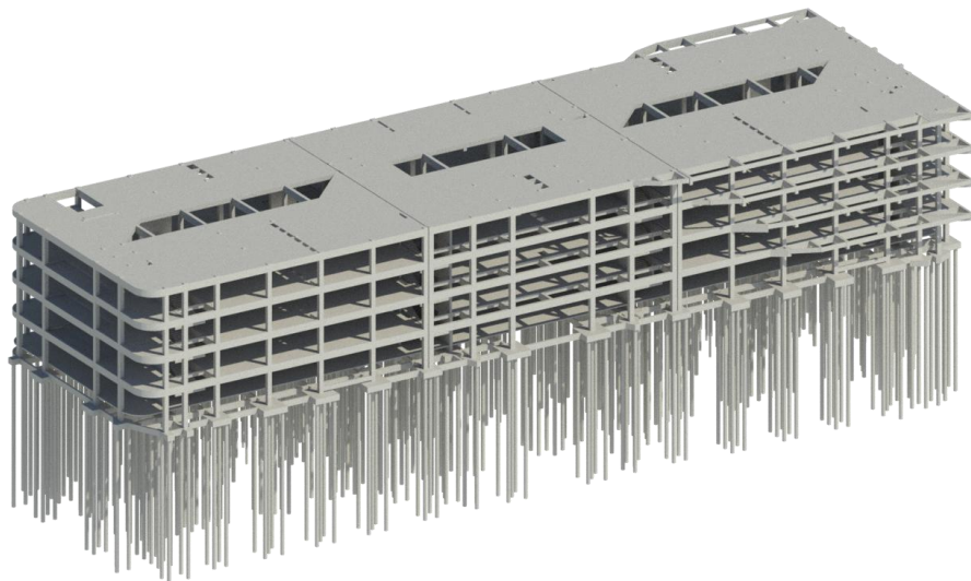
公共教学楼主体结构 BIM 模型
