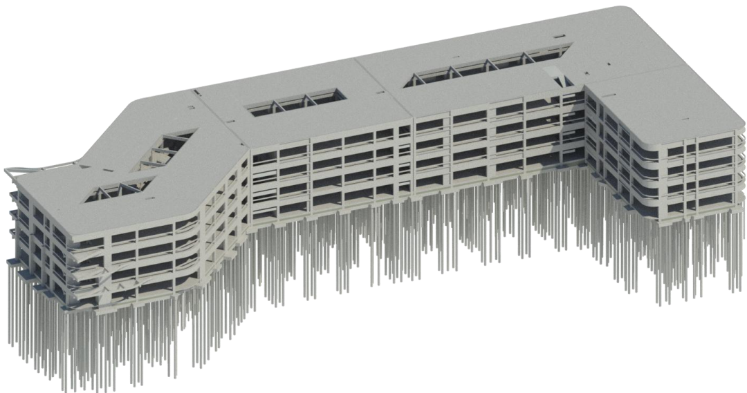
乘务飞行大楼主体结构 BIM 模型
