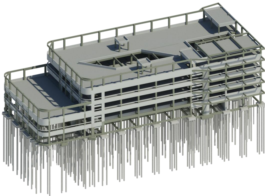
机场学院教学实验楼主体结构 BIM 模型
