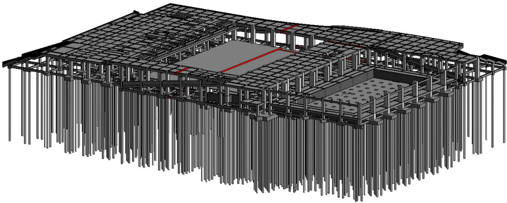
体育馆 BIM 模型
