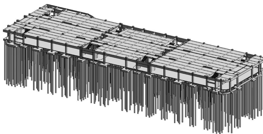
公共教学楼 BIM 模型
