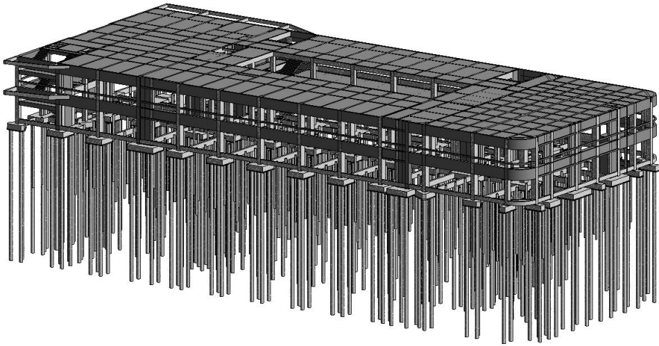
机场科学教研楼 BIM 模型
