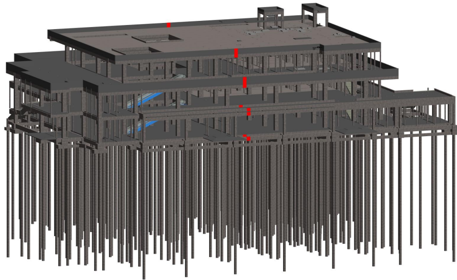
食堂（能源站）主体结构 BIM 模型
