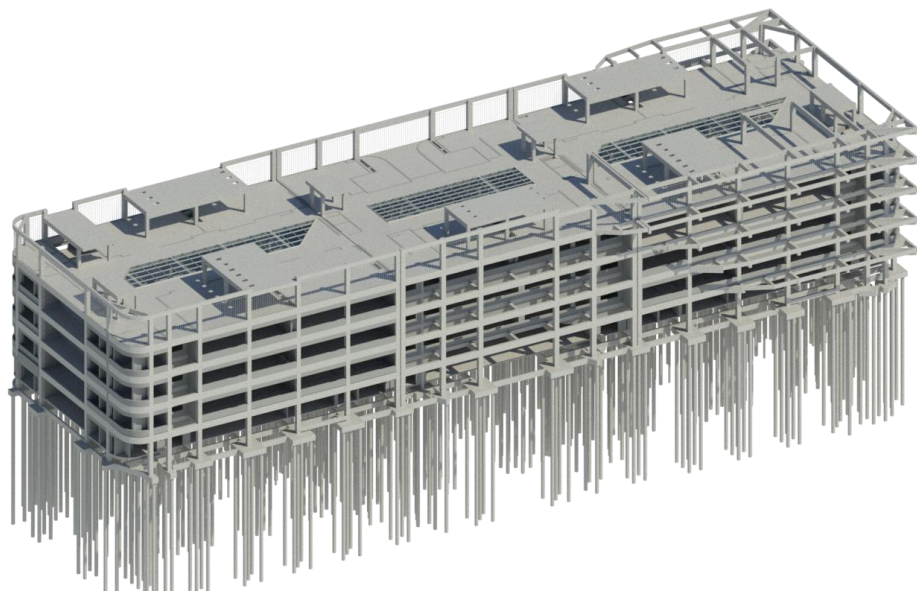
公共教学楼主体结构 BIM 模型
