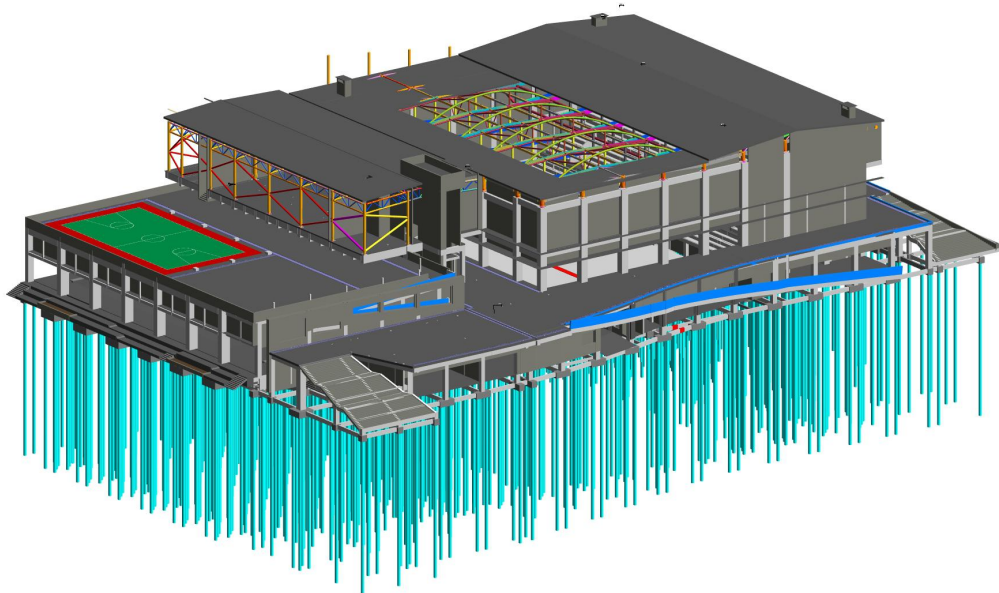
体育馆主体结构 BIM 模型
