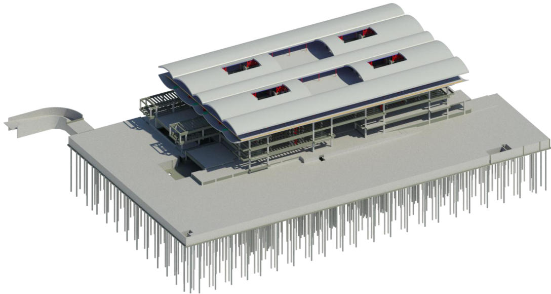
图书馆 BIM 模型
