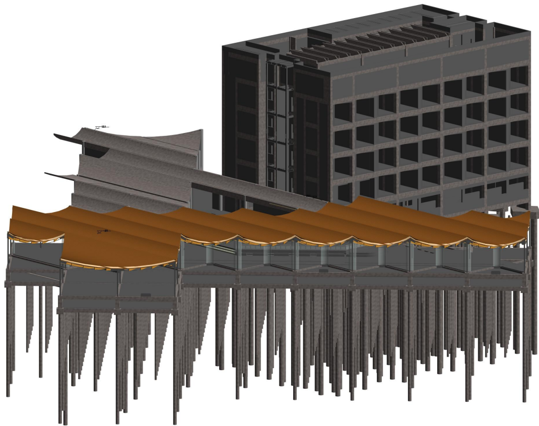
师生活动中心屋面施工完成，全面展开外墙保温施工。
