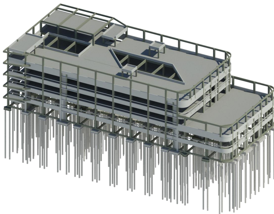
机场学院教学实验楼主体结构 BIM 模型
