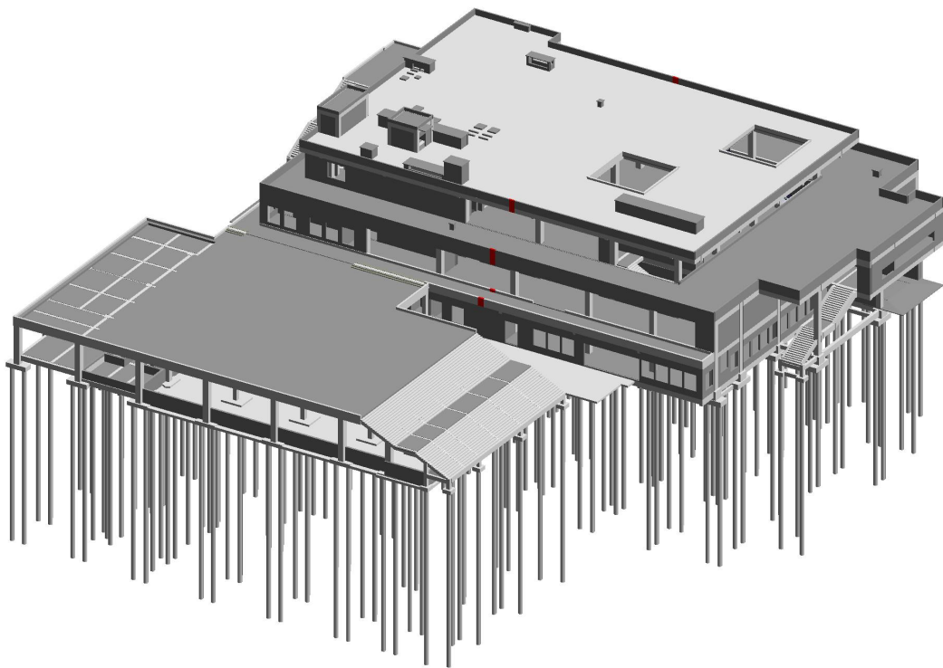
食堂（能源站）主体结构 BIM 模型
