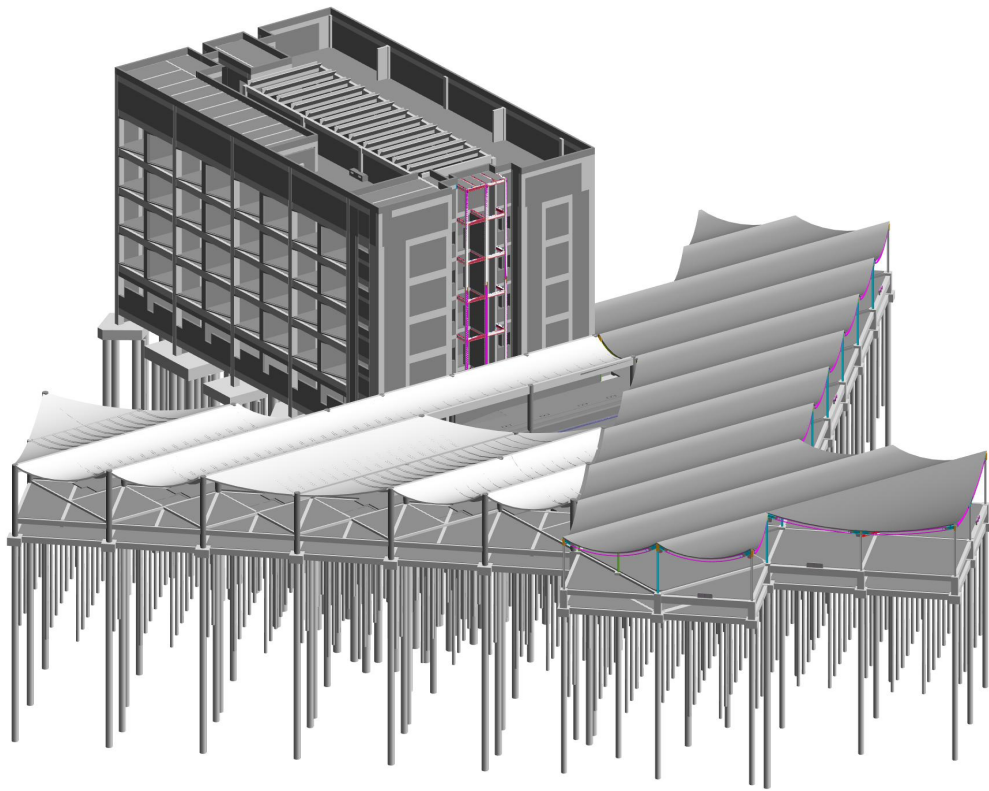
师生活动中心主体结构 BIM 模型
