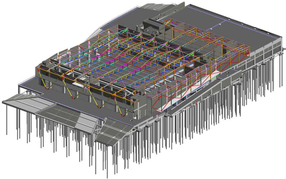
体育馆主体结构 BIM 模型
