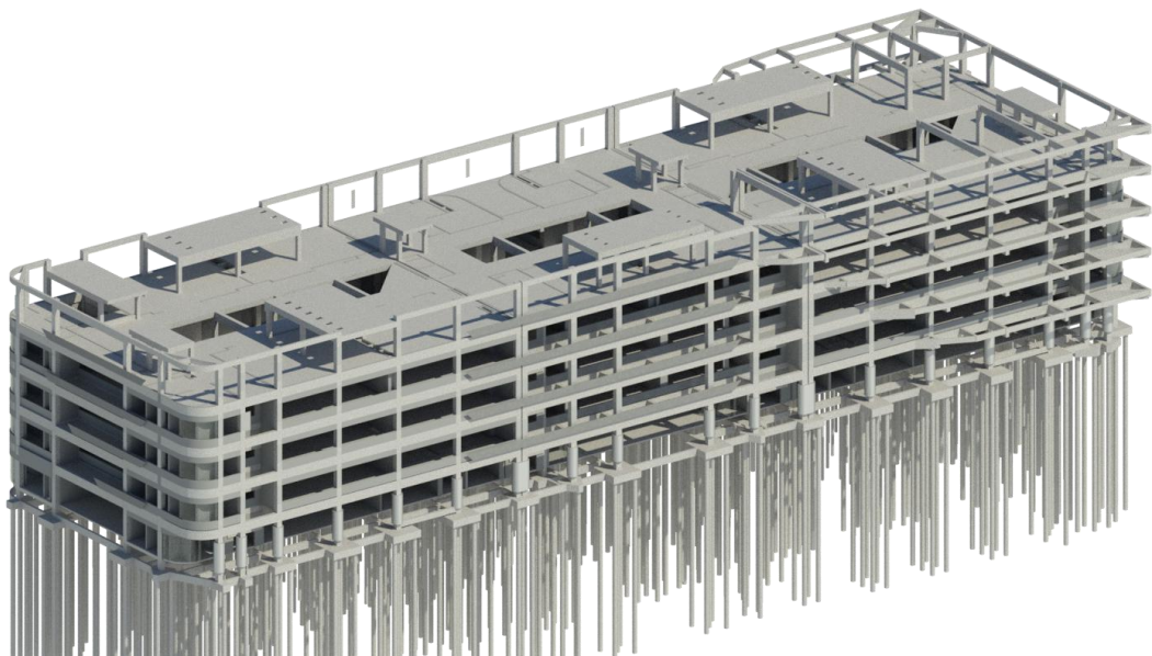
公共教学楼主体结构 BIM 模型
