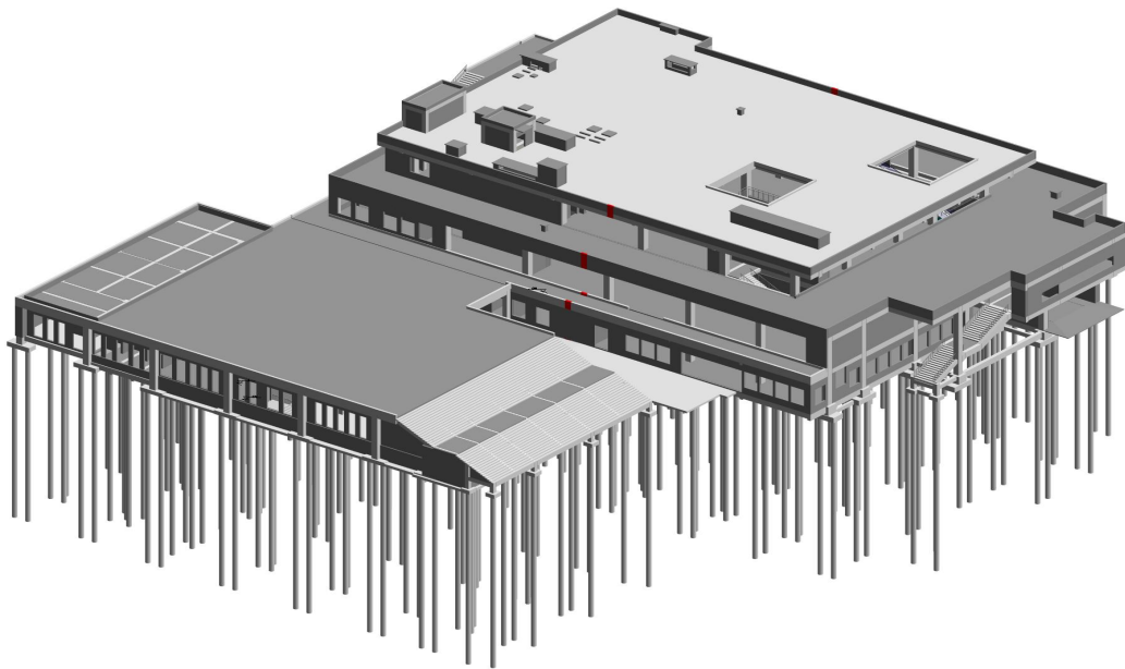
食堂（能源站）主体结构 BIM 模型
