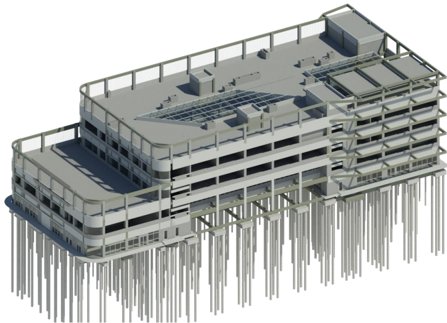
机场学院教学实验楼主体结构 BIM 模型
