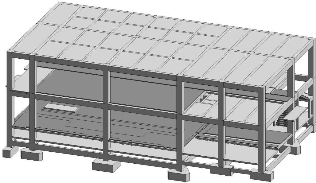
35KV 变电站主体结构施工完成
