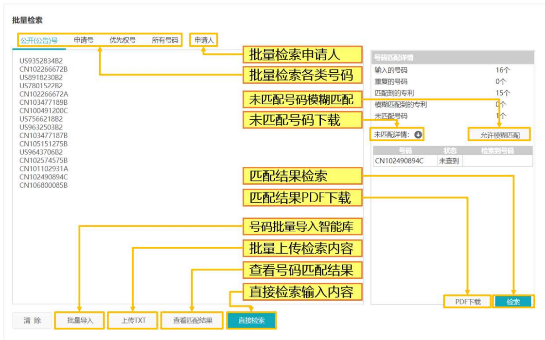
图 2-6 批量检索界面
