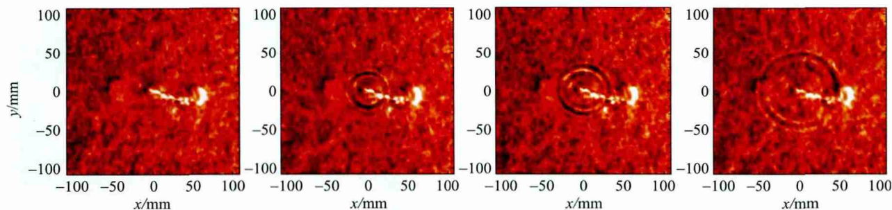
图3 1996年7月9日X2.6级耀斑引起的日震, 据称烈度相当于11.3级的地震, 由欧洲航天局(ESA)和美国国家航空航天局(NASA)联合研制的太阳和太阳风层探测器(Solar and Heliospheric Observatory, 缩写为SOHO) SOHO/MDI观测到。图中显示的是视线方向上(即垂直纸面)的速度场, 从中可以清楚的看到震波的传播。该结果取自 Kosovichev 和 Zharkova 在1998年 Nature 杂志上发表的文章 [7]
