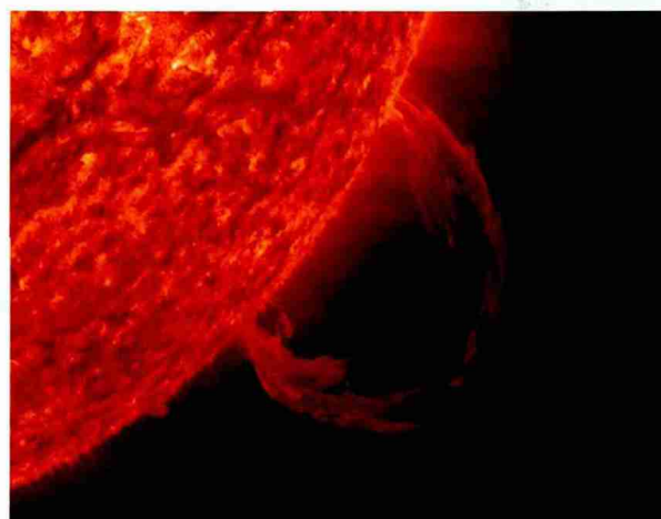
图2 2013年5月NASA太阳动力学天文台(SDO)观测到的一个太阳爆发事件中被抛出的等离子体磁绳(flux rope)
