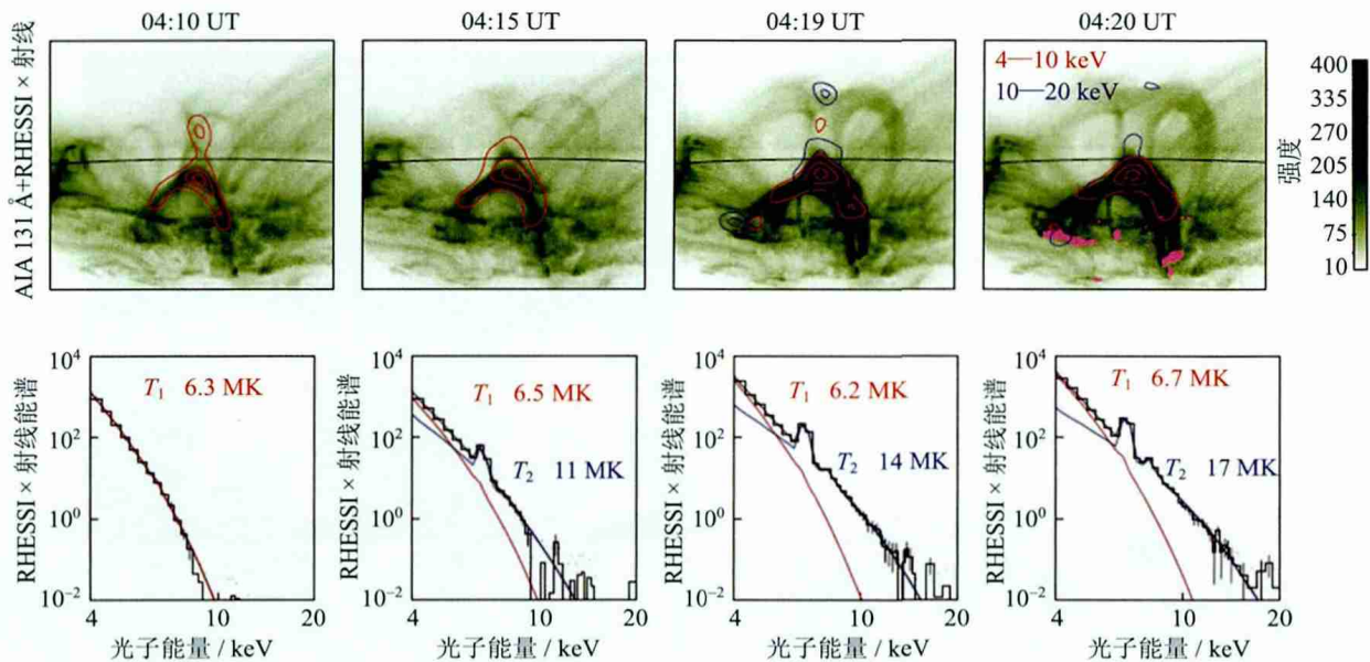
图7 上面的图显示不同时刻(国际时间)SDO/AIA观测到的热环和RHESSI观测到的X射线源(等值线)。图中粉红色标示出了日面上被加热的区域,它们对应于耀斑环的足点区。下面的图显示了RHESSI观测到的X射线能谱。通过对其进行双温度拟合得到两个热辐射分量,分别对应两个温度的等离子体(由红色和蓝色标出)。本图取自Su等人的文章 [14]
