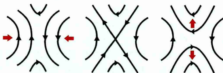
图5 磁场重联的示意图。相反走向的磁力线相互靠近，形成X型结构，重新连接后的磁场从另外两端像绷紧的皮筋一样弹出重联区。取自文献 [10]
