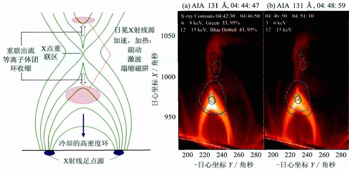
图8 左侧显示了一个太阳爆发的磁重联示意图; 右侧的两幅图像显示的是SDO/AIA所观测到的磁重联, 包含热耀斑环、尖角状结构以及X射线源(等值线, 由RHESSI成像得到)。X和Y表示日心坐标系东西和南北方向上距离日面中心的距离。其中1角秒对应太阳上700多千米。该图取自Liu等人的文章 [26]
