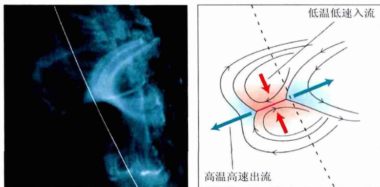
图6 Terry Forbes在其评论文章 [20] 中对Su等人研究的太阳爆发所做的图解。左侧是AIA 131 Å的观测, 右侧是磁场重联的示意图。红色箭头代表相对低温的入流, 蓝色箭头代表高温出流, 红线代表中间的电流片
