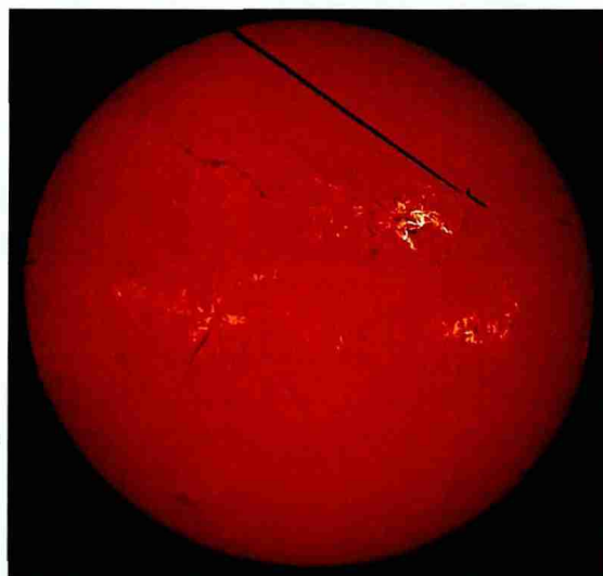
图1 一架飞机掠过H-alpha望远镜中的太阳表面。飞机左侧的亮带是一个活动区内被耀斑所加热的表层大气。图中狭长的暗带是暗条,而活动区内黑色的斑状结构是黑子。该图由奥地利格拉茨大学Kanzelhöhe天文台提供
