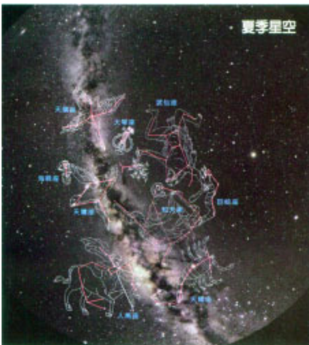
绘有星座轮廓的夏夜星空照片
