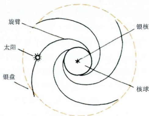
银河系结构示意图(上)侧视(下)俯视
