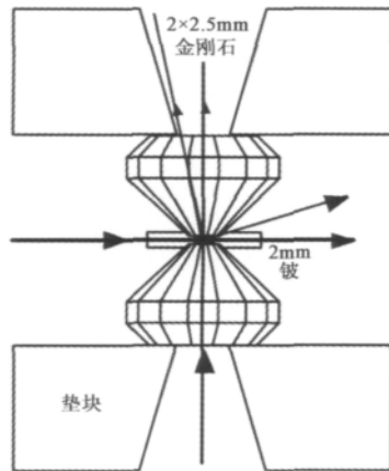
图4 对金刚石压砧中的样品,同步辐射 X 射线可以有不同入射方式,这里显示的有正入射和侧入射两种
