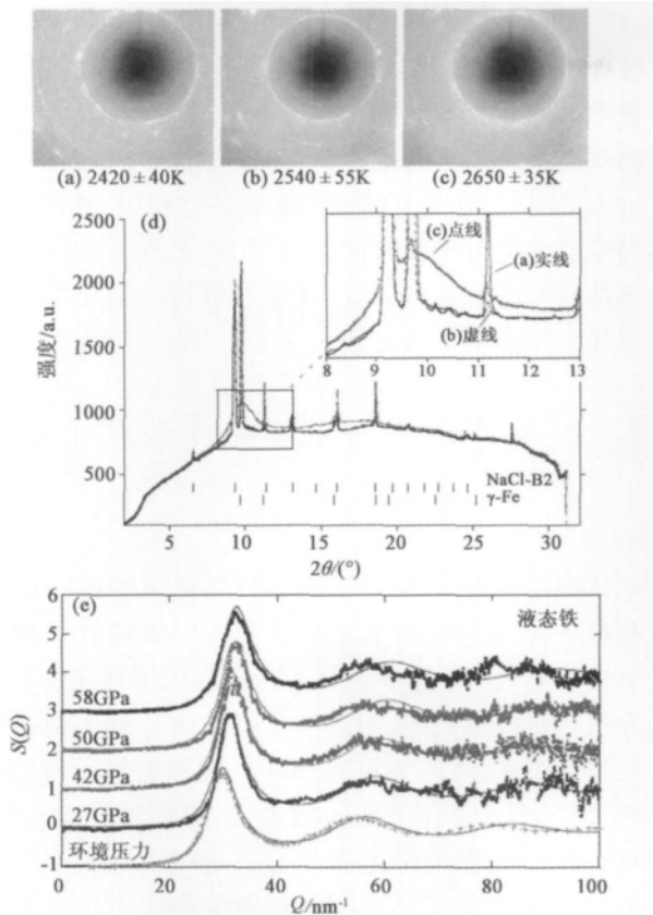
图6 在50GPa的高压下铁的X射线衍射图谱(a)和(b)为未熔化时不同温度下固态铁的衍射图像记录;(c)熔化后液态铁衍射图像记录;(d)由上述衍射图像记录综合的衍射图谱;(e)由高压X射线散射所确定的液态铁的结构因子 S 与散射动量 Q 的关系曲线
