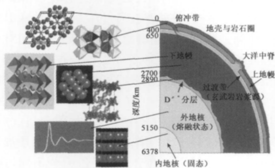
图7 通过高温高压实验,人们目前对地球内部的物质组成和状态有了较深入的了解.例如,在板块俯冲带可能出现从橄榄石到尖晶石的相变;下地幔的主要矿物是钙钛矿;在核幔边界的超低速带,钙钛矿进一步转变成超钙钛矿;地核分为液态的外地核和固态的内核,其主要组分是铁,并含有少量其他轻元素(如Si和S等)
