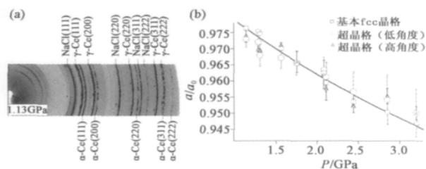
图3 利用北京电子对撞机同步辐射装置高压光束线较低能量(17keV)的单色 X 射线,通过高压 X 射线衍射实验,我们在低衍射角(2.2°—3.5°)的区域中观察到了疑似 \alpha -Ce 对称破缺的超晶格结构(a)压力为 1.13GPa 时观测到的原始二维 XRD 衍射图,其中最左侧低衍射角位置的 4 条较弱的衍射峰即为疑似超晶格的衍射峰,而标记为 NaCl 的衍射峰来自样品周围作为压力标准与传压介质的 NaCl;(b)超晶格的平均压缩比( a/a_0 )随压力的变化与基本 fcc 晶格压缩比随压力的变化的比较.可以看到,在实验误差范围内,高、低衍射角位置的衍射峰所代表的超晶格与 \alpha -Ce 的基本 fcc 晶格的压缩比随压力的变化基本一致,即它们有相同的状态方程.同时可以看到,超晶格结构的压缩比具有较大的误差,除了因为衍射强度相对弱外,根据衍射理论分析,相当低的衍射角应该是误差较大的主要原因
