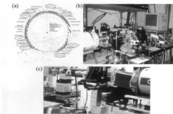
图 1 同步辐射装置中的高压实验站照片 (a) 美国芝加哥的 Argonne 国家实验室的先进同步辐射光源 (APS). 除了高压专用的 HPCAT 和 GeoCARS 之外,还有其他 11 个光束线都结合了高压技术,可以开展静高压实验研究工作(带圈标记的线站);(b) 北京正负电子对撞机同步辐射装置高压实验站, X 射线束由右向左入射;(c) Brookhaven 国家实验室 NSLS 的 X17C 高压实验站, X 射线束由左向右入射
