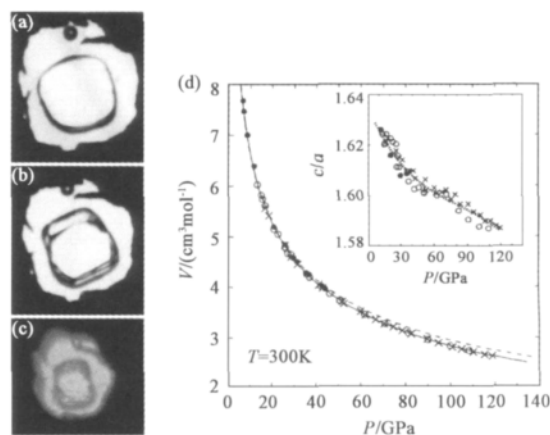
图 2 氢和氘的状态方程. 左图为在金刚石压砧中以氘为传压介质制备的单晶氘, 图(a)、(b)、(c)分别是单晶氘在 10GPa、14GPa 以及 119GPa 高压下的照片; (d)为测得的状态方程(压力 P 和比容 V 的关系)
