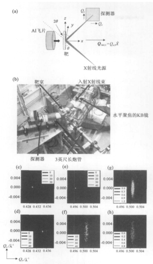
图8 在美国芝加哥的 Argonne 国家实验室的先进同步辐射光源 (APS) 的高压专用束线与实验站 HPCAT, 首次成功地尝试了冲击压缩 X 射线衍射实验。(a) 和 (b) 分别为冲击压缩实验的实验设计原理图和实验装置照片; (c) — (h) 为实验结果的倒格子空间衍射图样。实验样品分别为纯的和镁掺杂的氟化锂单晶; (c) 和 (d) 分别表示纯氟化锂单晶在冲击前和冲击中的衍射图样; (e) 和 (f) 分别表示镁掺杂的氟化锂单晶在冲击前和冲击中的衍射图样; (g) 和 (h) 分别表示采用两种不同的结构参数对图 (f) 实验结果的数值模拟
