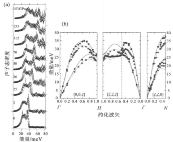
图5 利用 X 射线的非弹性散射测得的铁和钨的晶格振动谱 (a) 利用穆斯堡尔效应测得的铁在 150GPa 时的晶格振动谱; (b) 在 17GPa 时钨的声子色散关系(其中实心符号代表非弹性 X 射线散射测量结果,空心符号代表非弹性中子散射测量结果,圆形符号代表纵声学模,方块代表横声学模.沿 (\xi, \xi, 0) 方向的三角与方块分别表示 2 个非兼并的横声学模 \text{TA}[110]\langle -110 \rangle 和 \text{TA}[110]\langle 001 \rangle )
