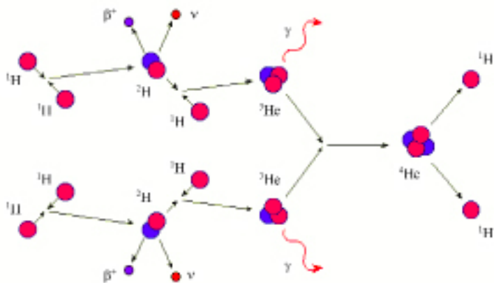
图3 氢燃烧的 pp 链反应
