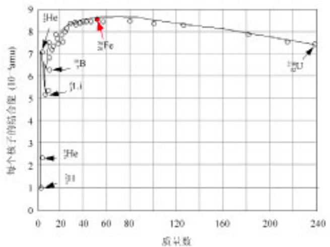
图8 元素的结合能
