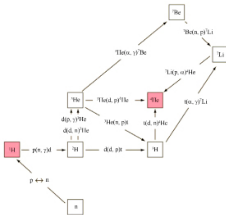
图 1 原初核合成的反应过程。其中 \gamma 为光子、 p 为质子、 n 为中子、 d 为氘、 t 为氚、 \alpha 为氦
