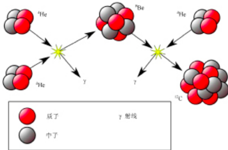
图4 氦燃烧的核反应
