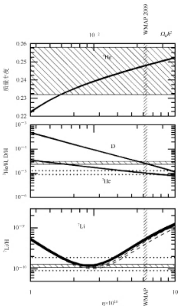
图2 原初元素的丰度。其中横坐标 \eta 是重子数和光子数之比，纵坐标从上到下分别是氦的质量丰度、氦3和氘核的数密度、锂核的数密度（与氢核的数密度之比）。此外， \Omega_b 是重子能量密度与特征能量密度之比， h 是约化哈勃常数。图中水平的阴影和虚线为实测数据所给出的范围，竖直的阴影是宇宙微波背景卫星 WMAP 所给出的测量结果
