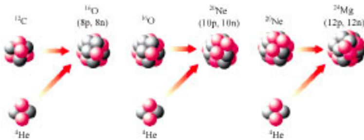
图5 核合成的 \alpha 过程
