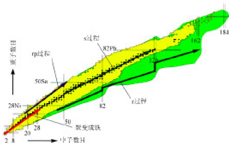
图9 元素核合成的主要过程
