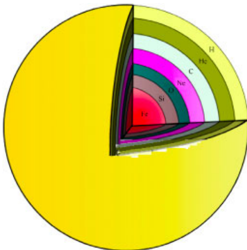
图7 超新星爆发前的恒星核心
