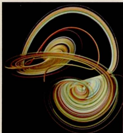
图3 数值模拟的地磁场磁极方向在天文学时间尺度下无规则的翻转
