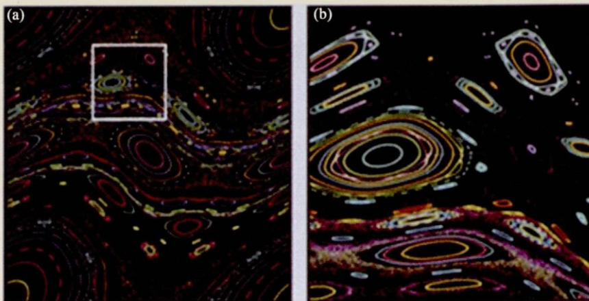
图2 (a) 周期驱动转子相空间轨迹的频闪映射，闭合环对应于周期和准周期运动区域，散点对应于混沌运动；(b) 图(a)中白框的放大，显示出自相似性
