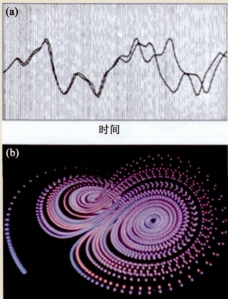
图 1 (a) Lorenz 从差别细微的两个初始条件演化得到的时间序列原始数据；(b) Lorenz 吸引子。Lorenz 方程为： dX/dt = \sigma(-X + Y) ， dY/dt = rX - Y - XZ ， dZ/dt = -bZ + XY ，其中 X 代表对流运动强度， Y 正比于上升与下降流的温差， Z 刻画对垂直方向温度分布的线性偏离， \sigma 为 Prandtl 数， b 为几何参数， r 为瑞利数
