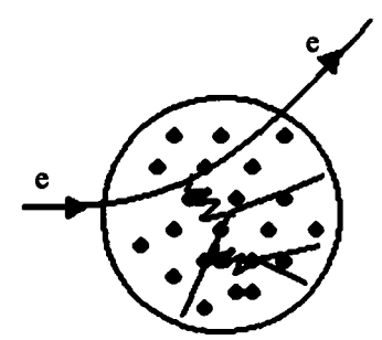
图5 电子-质子深度非弹性散射
