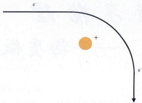
图3 电子在质子上的散射
