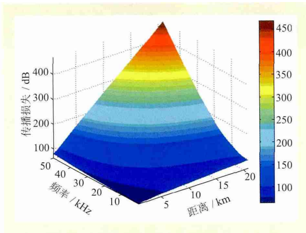
图3 传播损失与距离和频率的关系示意图
