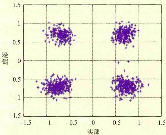
图9 均衡器输出星座图
