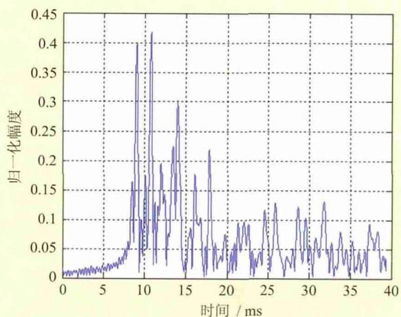
图6 2007年1月渤海4 km实测信道
