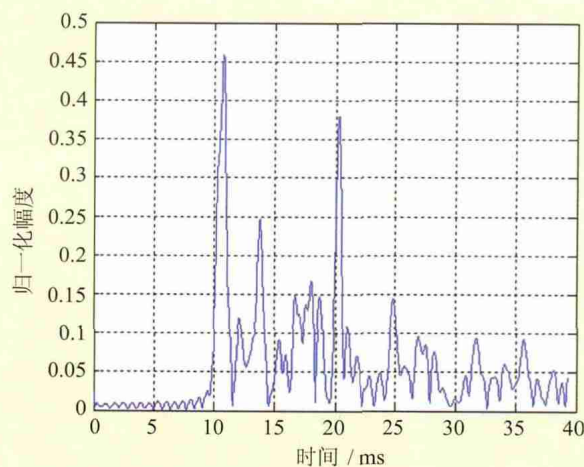
图5 2005年4月东海1 km实测信道
