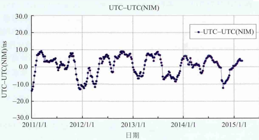
图2 协调世界时UTC与中国计量院(NIM)地方协调时UTC(NIM)之差
