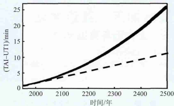
图4 预测原子时TAI与天文时UT1之差(实线表示地球转速在“正在变慢”;虚线表示地球转速比以前“慢了”)
