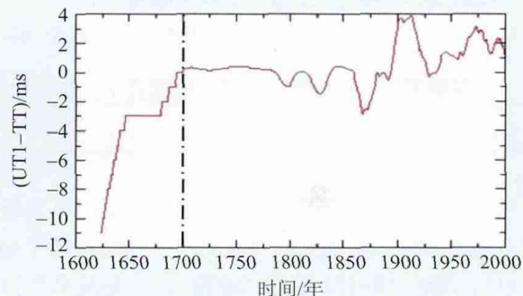
图5 天文时与地球原子时之差UT1 - TT(其中UT1为天文时,TT为地球时,是国际原子时的平均值)
