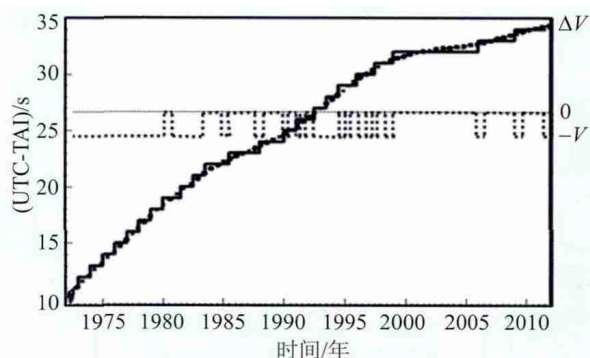
图3 1972年至今的闰秒记录(图中虚线和右边纵坐标表示地球自转相对速率波动)
