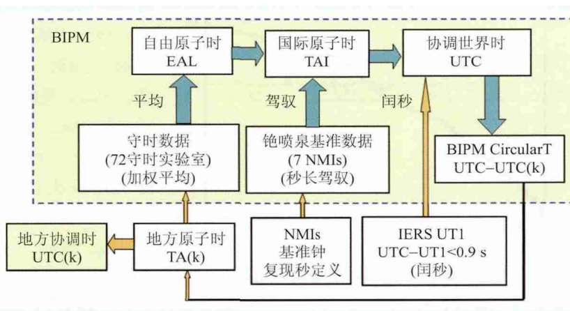
图1 国际原子时合作产生协调世界时(UTC)(图中BIPM为国际计量局, Circular T为时间公报, NMIs为各计量院, IERS为国际地球自转局, UT1为世界时UT1)
